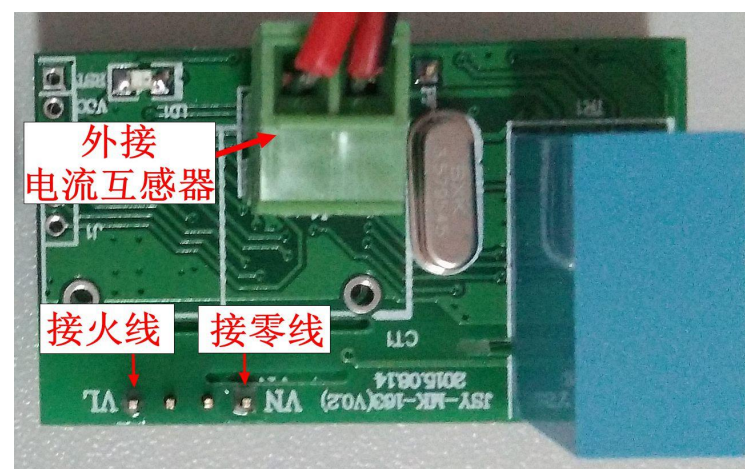
接线示意图
