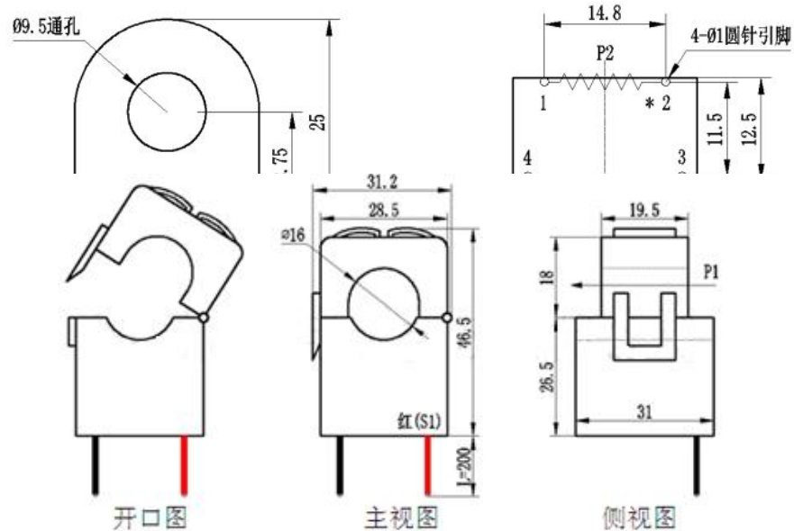
电流互感器外型及尺寸图:
